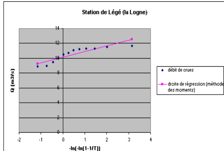
graphe 4: Méthode Gumbel sur la Logne, Legé
