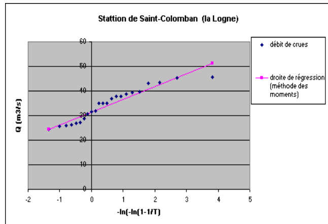
graphe 5: Méthode Gumbel sur la Logne, Saint-Colomban
