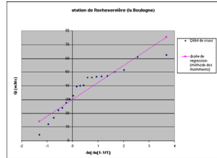
graphe 6: graphe 1: Méthode Gumbel sur la Boulogne, Rocheservière
