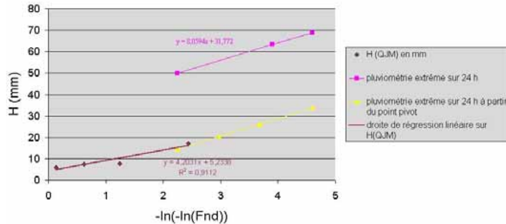
graphe 8: Méthode Gradex appliquée à la station de Legé
