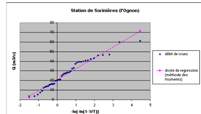
graphe 7: Méthode Gumbel sur l'Ognon, les Sorinières
